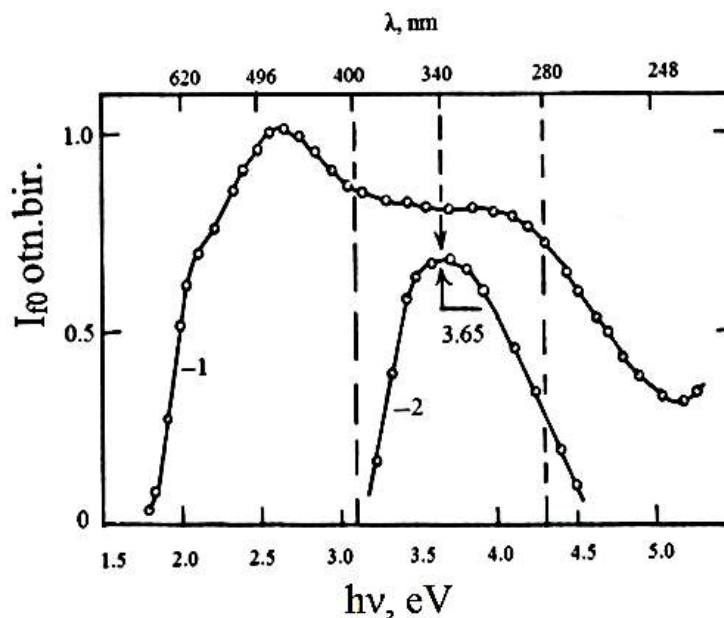
2-nji surat. Au-Ga 2 O 3 -n-GaAs 0,6 P 0,4 Şottki diodynyň fototogunyň giň diapozonyndaky spektri: (1), UFS-2 filtr bilen korrektirlenen fototogyň spektri (2) Fototogyň spektri deň sanly fotonlaryň düşüşine normirlendi
