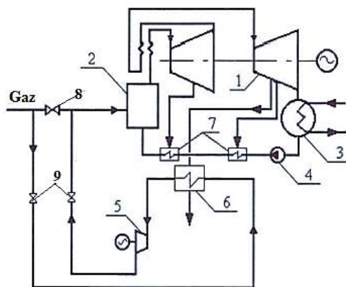
1-nji çyzgy. Energoblogyň ýylylyk shemasyna generatorly turbodetander desgasynyň birikdiriliş çyzgysy: 1 – turbina; 2 – gazan; 3 – kondensator; 4 – sorujy; 5 – detander; 6 – gazy gyzdyrmaga ýylylyk çalşyjy; 7 – regeneratiw gyzdyryjy
